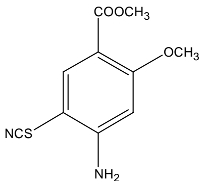
2-甲氧基-4-氨基-5-乙磺基苯甲酸甲酯
