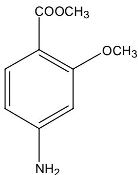
2-甲氧基-4-氨基-5-硫氰基苯甲酸甲酯
