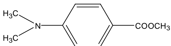
对二甲氨基苯甲酸甲酯
